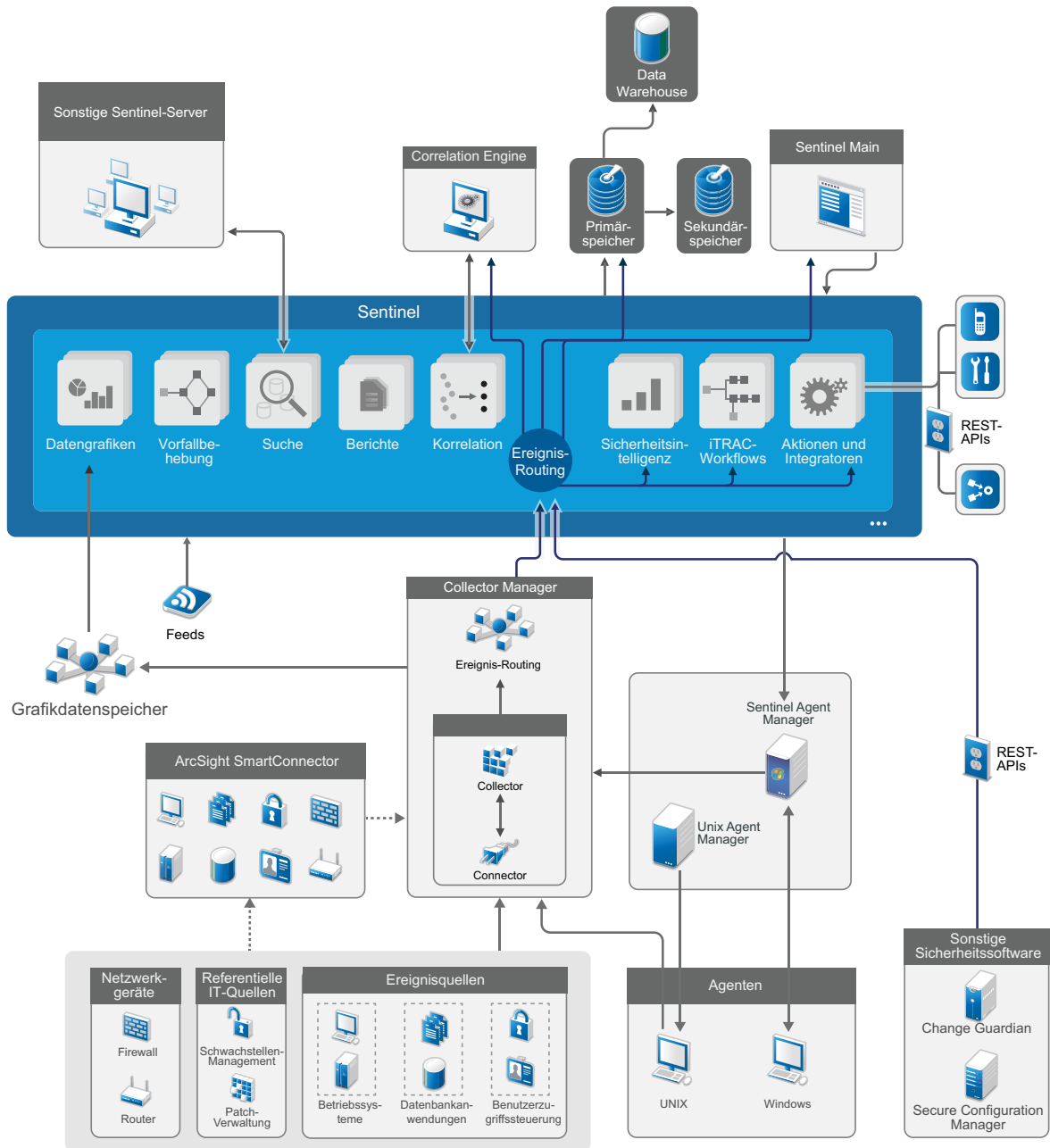
Abbildung 2-1 Sentinel-Architektur
