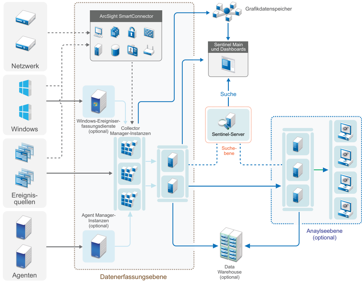
Abbildung 6-4 Verteilte Zwei-Ebenen- und Drei-Ebenen-Bereitstellung
