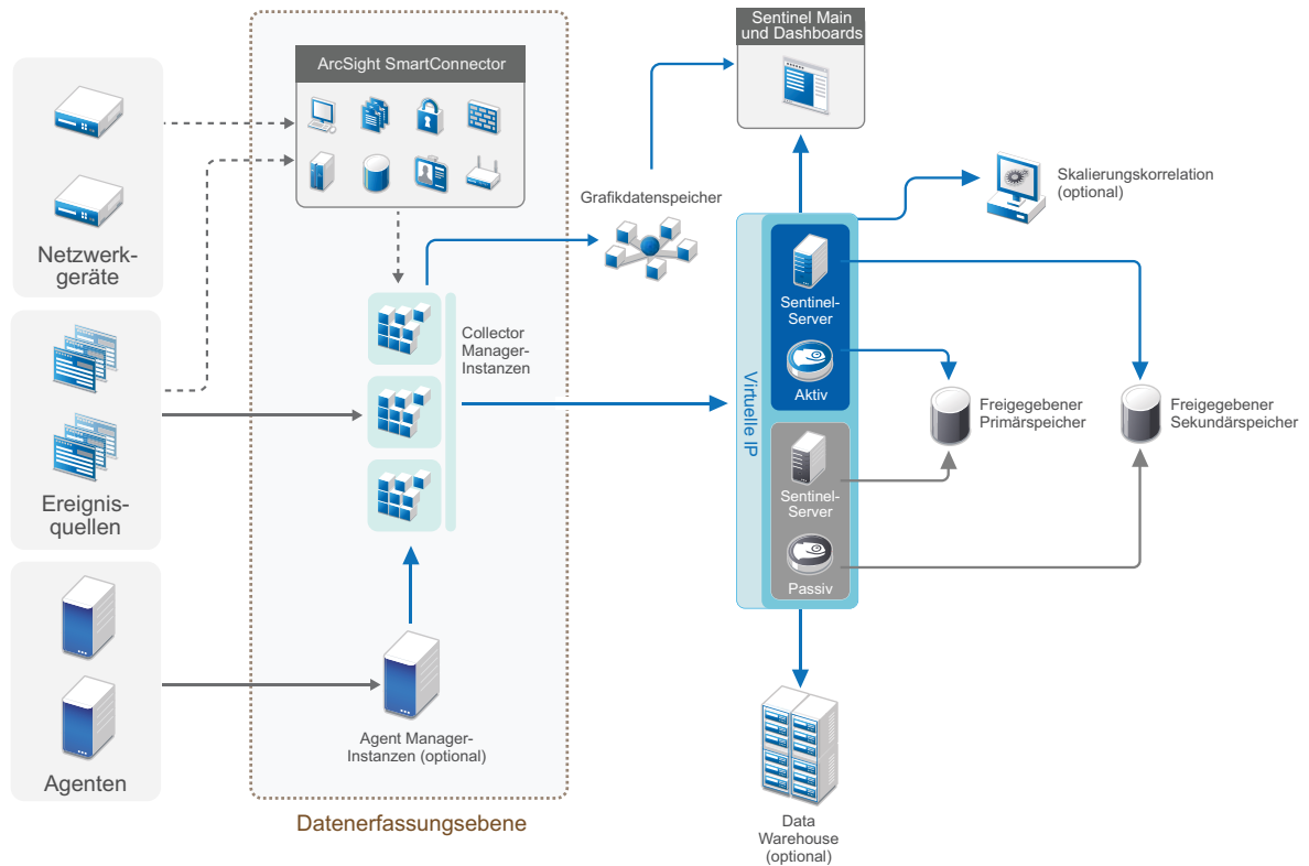
Abbildung 6-3 Verteilte Ein-Ebenen-Bereitstellung mit hoher Verfügbarkeit
