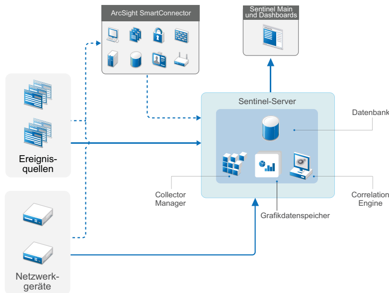
Abbildung 6-1 All-In-One-Bereitstellung
