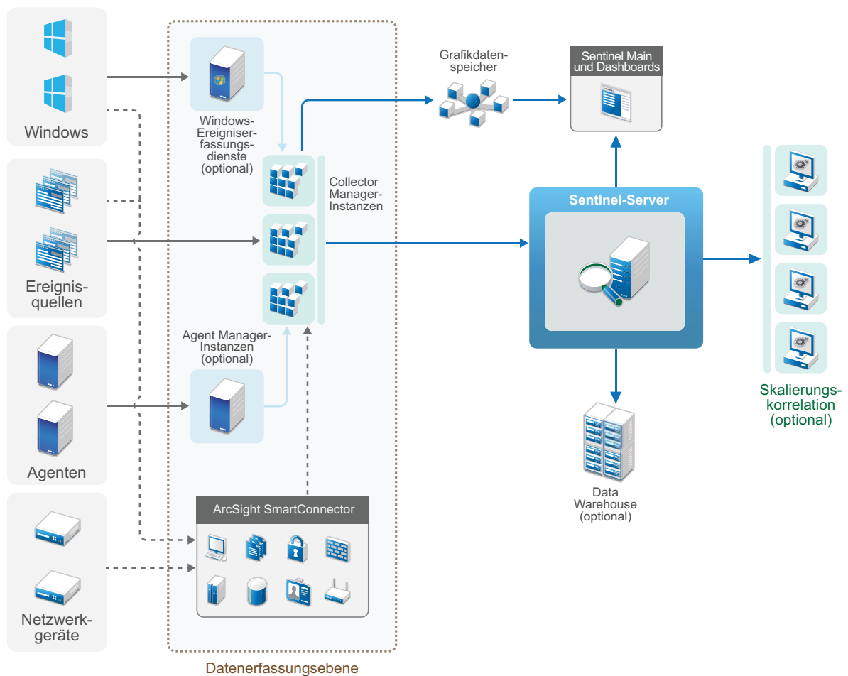
Abbildung 6-2 Verteilte Ein-Ebenen-Bereitstellung
