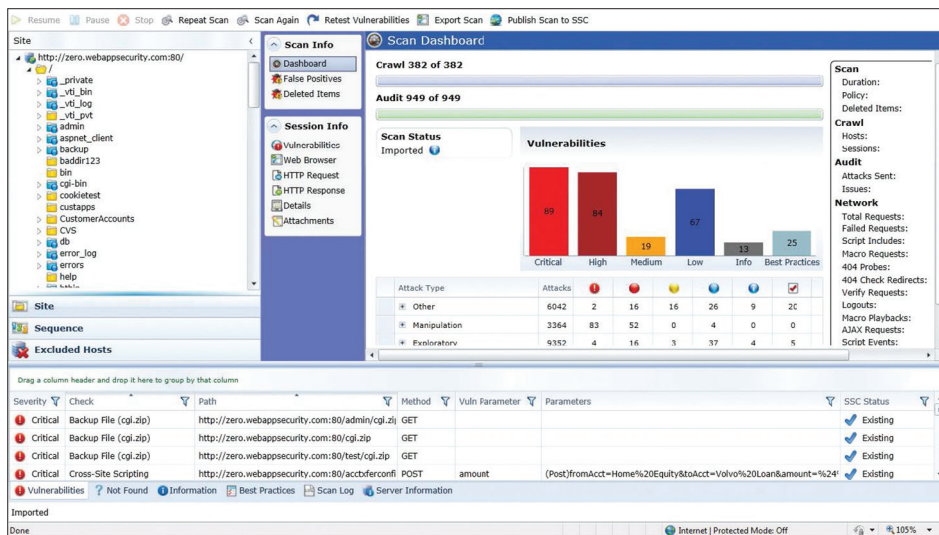
図 2 WebInspect Enterprise の Web ベース GUI
