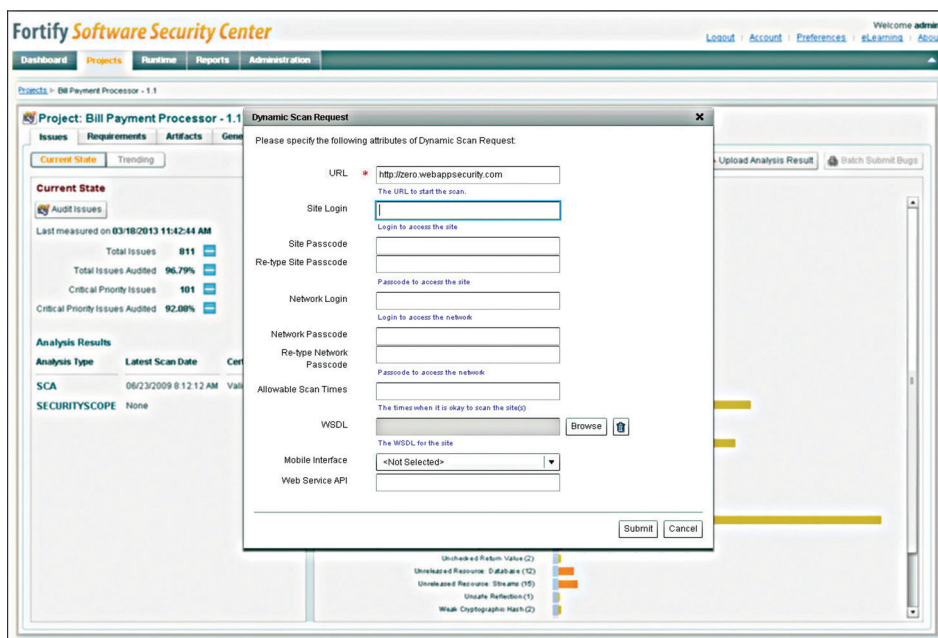
図 1 動的スキャン要求で評価ワークフロープロセスを大幅に改善
